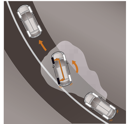
Programa de estabilidad electrónica (ESP).
